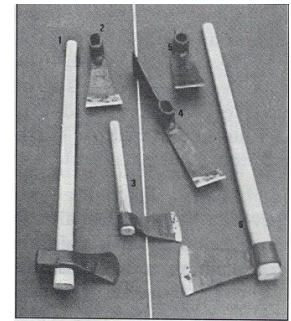
1 Merlin emmanché 2 Houe à défricher 3 Hachette emmanchée 4 Pioche - hache 5 Herminette 6 Hache œil ogival emmanché
